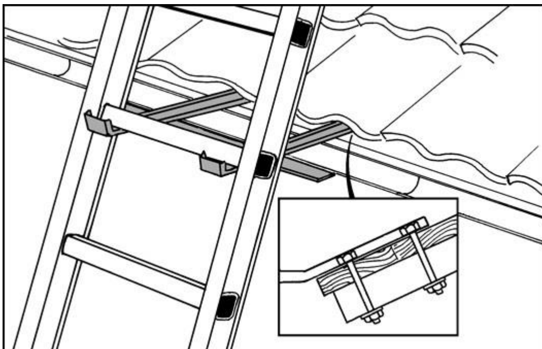
Teikning av montering av sklisikring.
